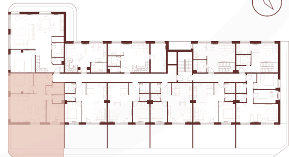
PÔDORYS PODLAŽIA
