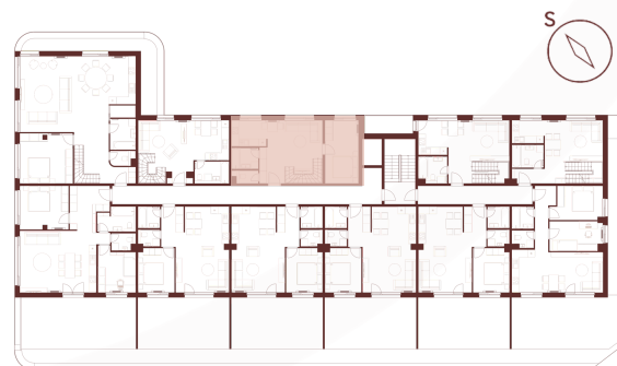
PŔDORYS PODLAŽIA
